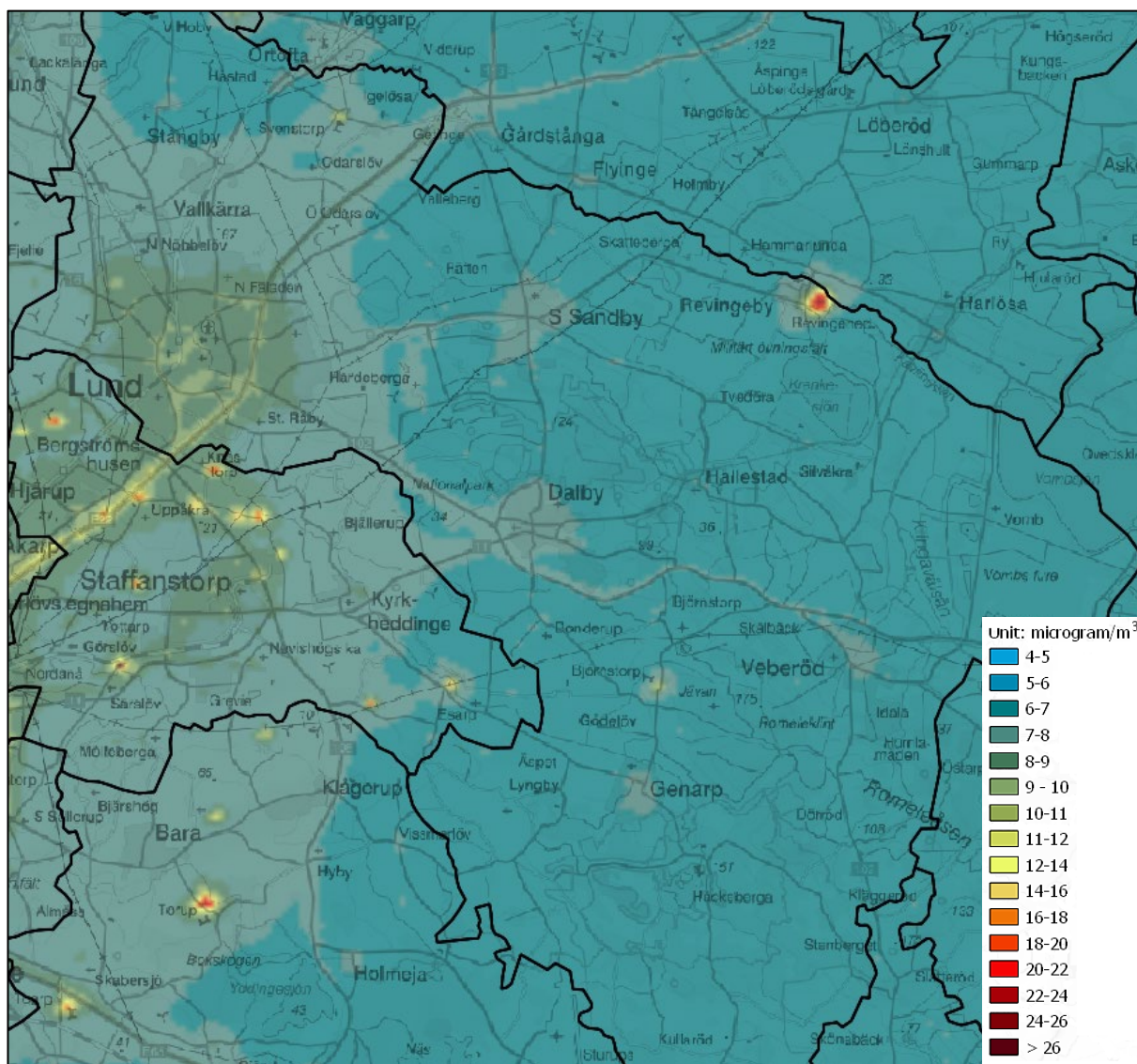
Figur 22. Beräknade årsmedelvärden av partiklar PM 2,5 inom kommunen (µg/m 3 ).
