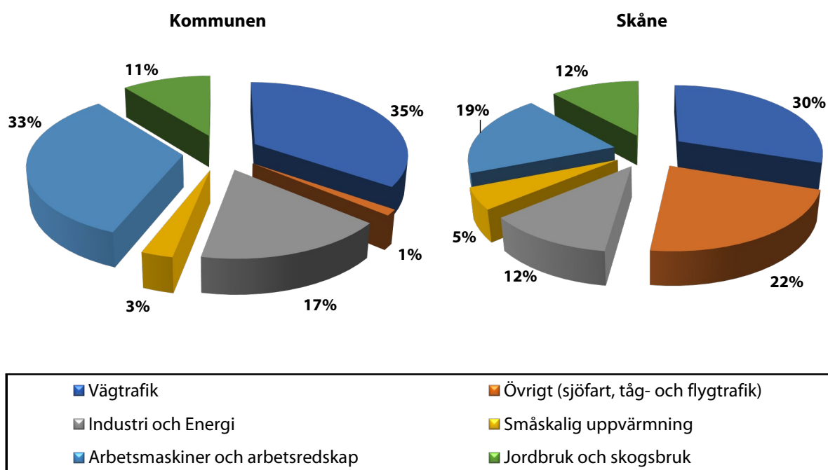
Figur 12. Procentuell fördelning av utsläppskällor för kväveoxider i kommunen jämfört med Skåne.
