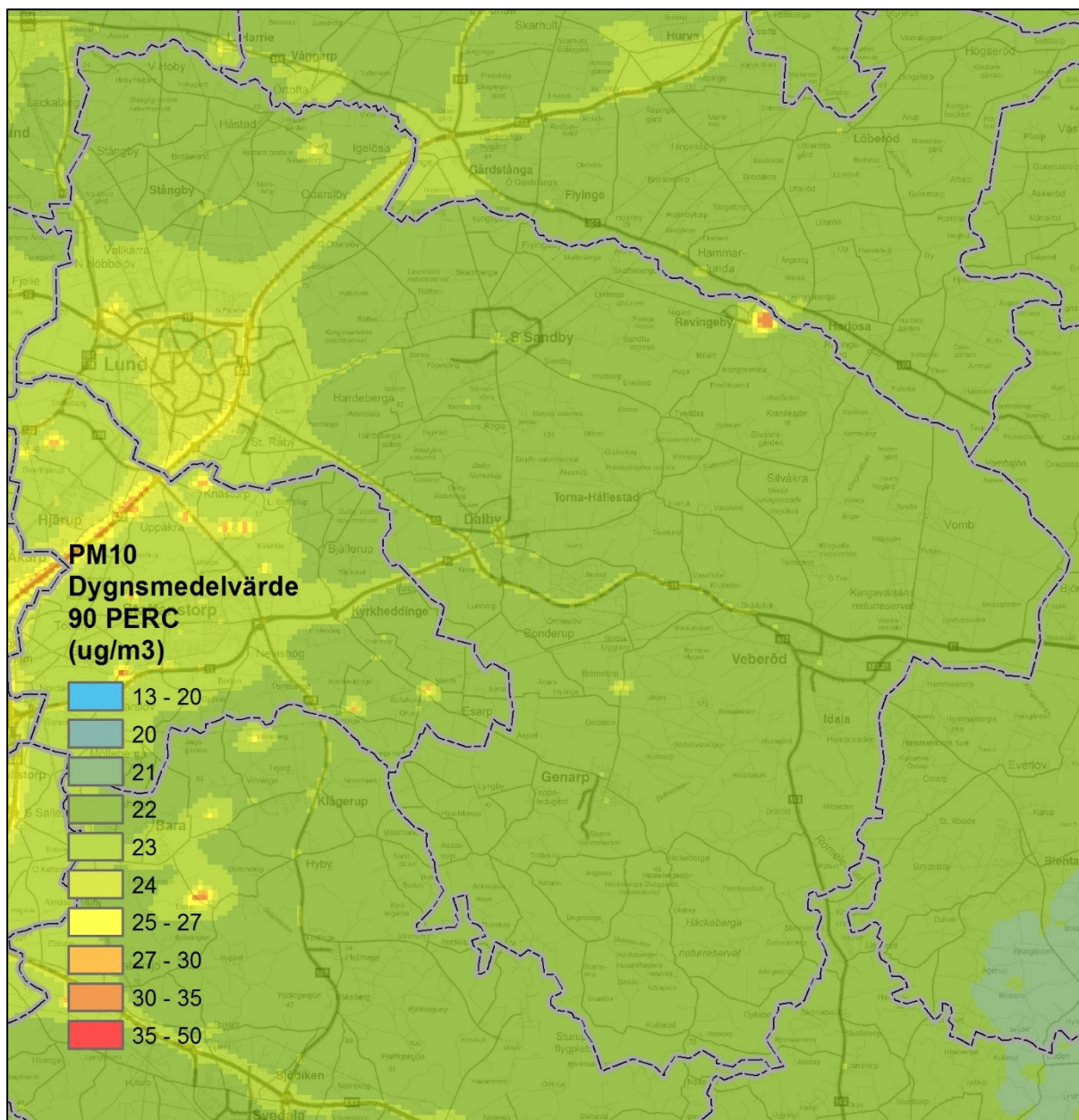
Figur 18. Beräknade dygnsmedelvärden av partiklar \text{PM}_{10} inom kommunen ( \mu\text{g}/\text{m}^3 ).
