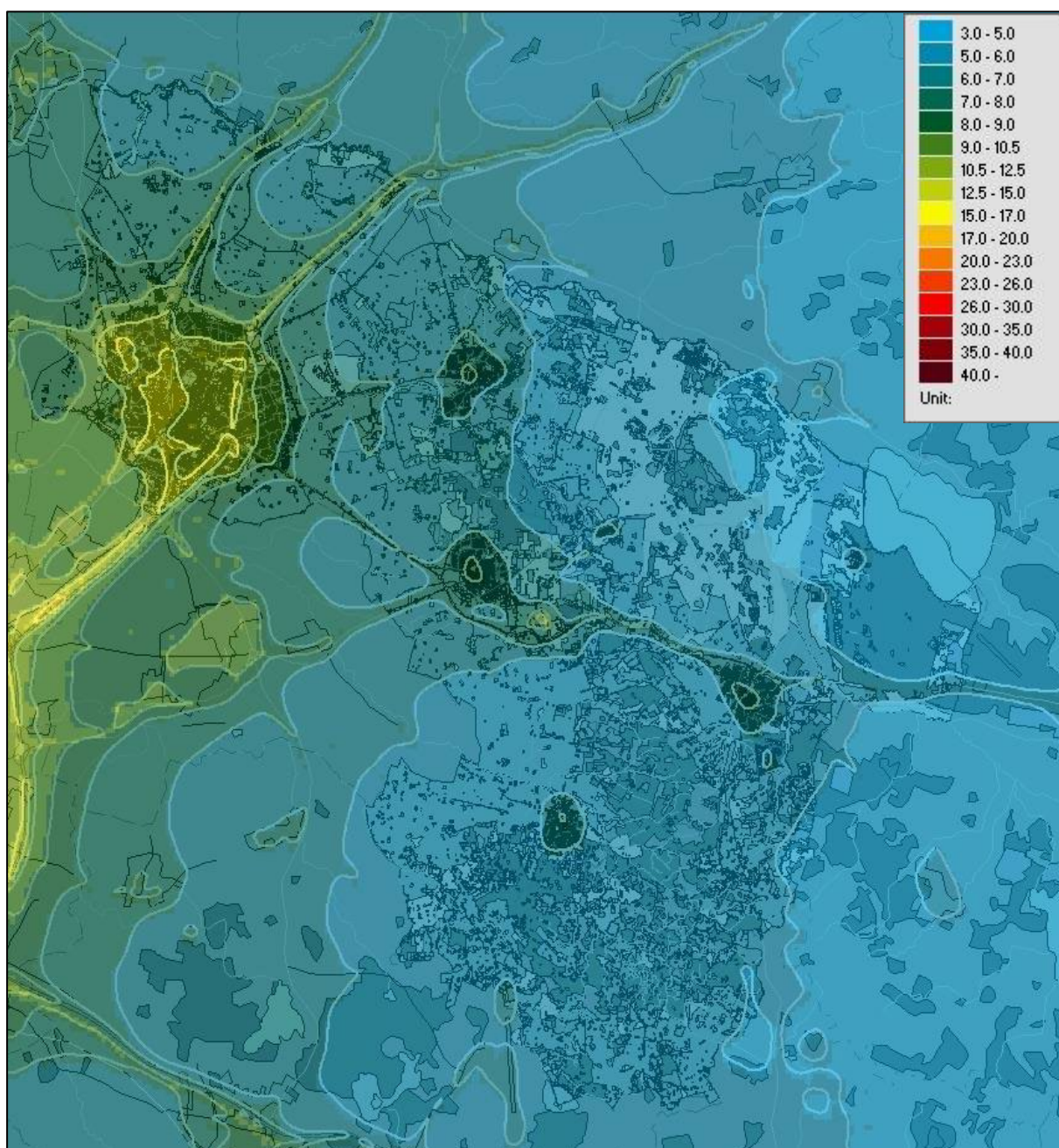
Figur 7. Beräknade årsmedelvärden av kvävedioxid inom kommunen ( \mu\text{g}/\text{m}^3 ).
