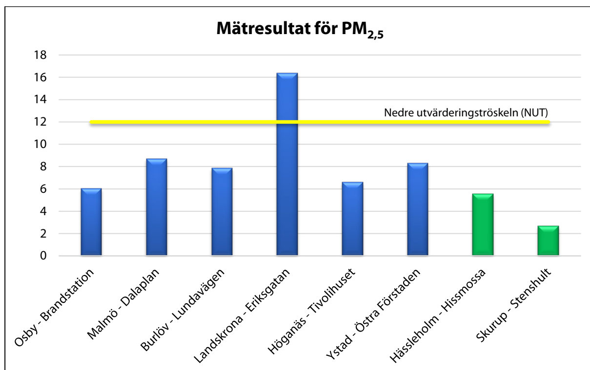
Figur 21. Medelvärde för partiklar (PM 2,5 ) under mätperioden inom samverkansområdet Skåne.
