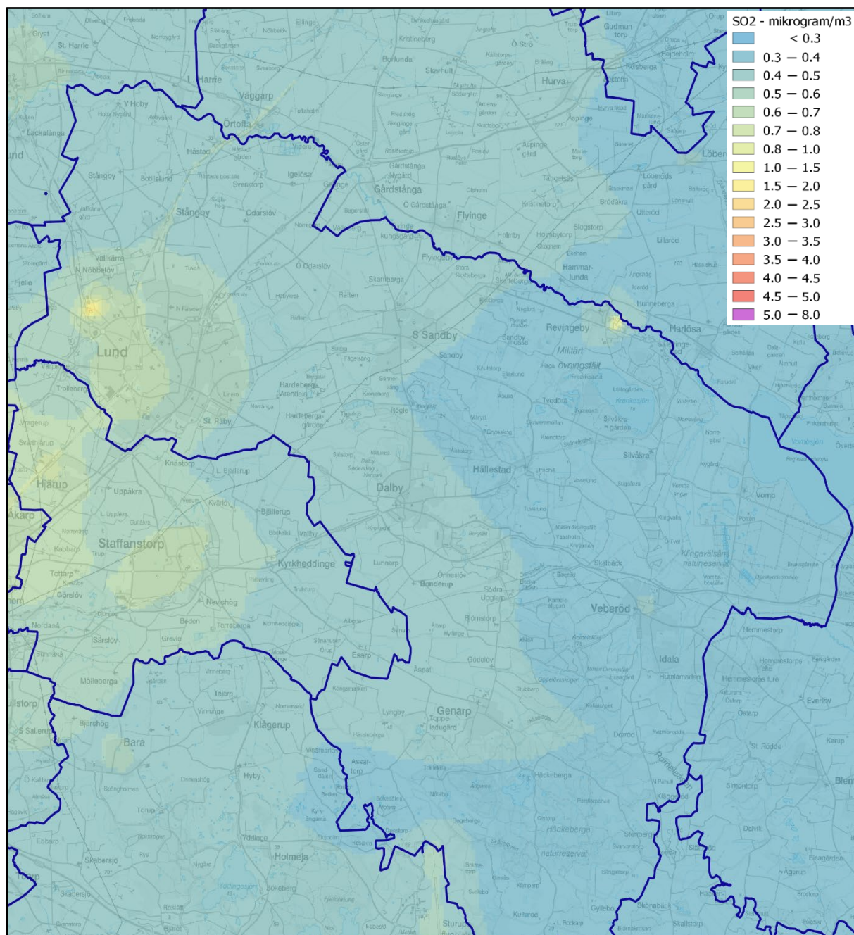
Figur 26. Beräknade årsmedelvärden av svaveldioxid ( \text{SO}_2 ) inom kommunen ( \mu\text{g}/\text{m}^3 ).
