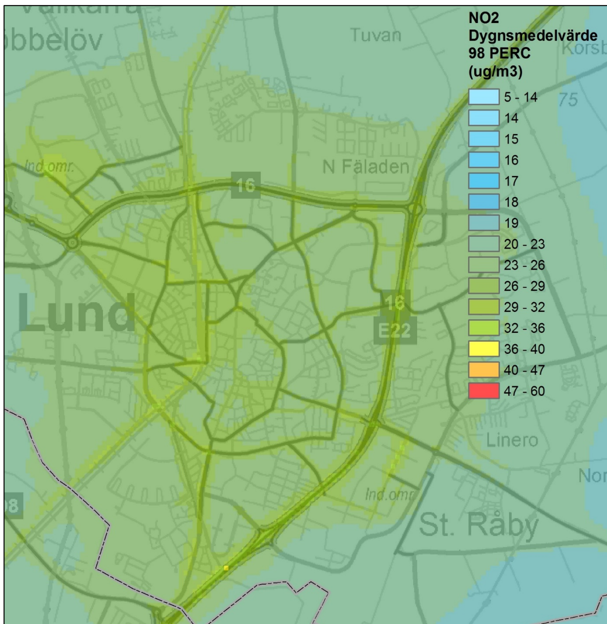
Figur 9. Beräknade dygnsmedelvärden av kvävedioxid i tätorten (µg/m³).
