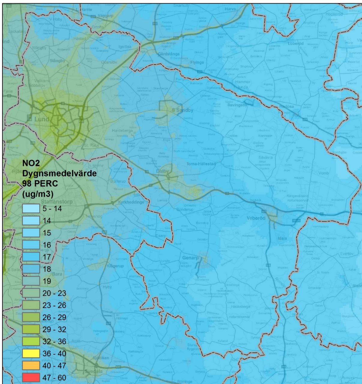
Figur 8. Beräknade dygnsmedelvärden av kvävedioxid inom kommunen ( \mu\text{g}/\text{m}^3 ).
