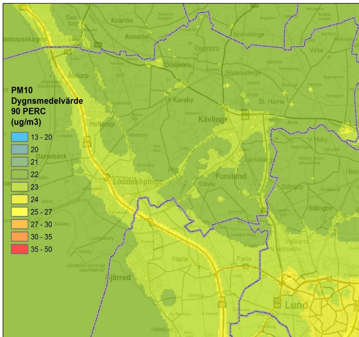
Figur 18. Beräknade dygnsmedelvärden av partiklar PM_{10} inom kommunen ( \mu\text{g}/\text{m}^3 ).
