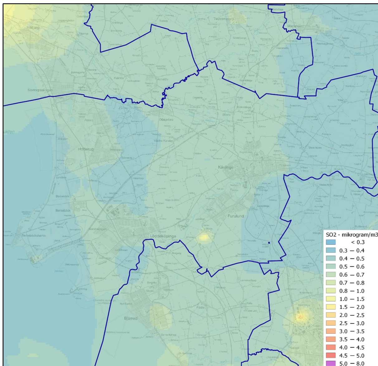
Figur 26. Beräknade årsmedelvärden av svaveldioxid ( \text{SO}_2 ) inom kommunen ( \mu\text{g}/\text{m}^3 ).
