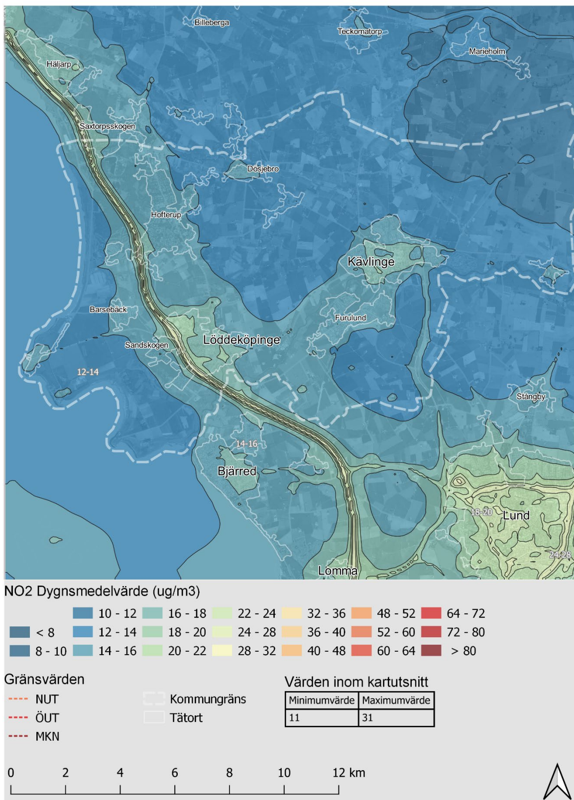
Figur 9. Beräknade dygnsmedelvärden av kvävedioxid inom kommunen (µg/m³).
