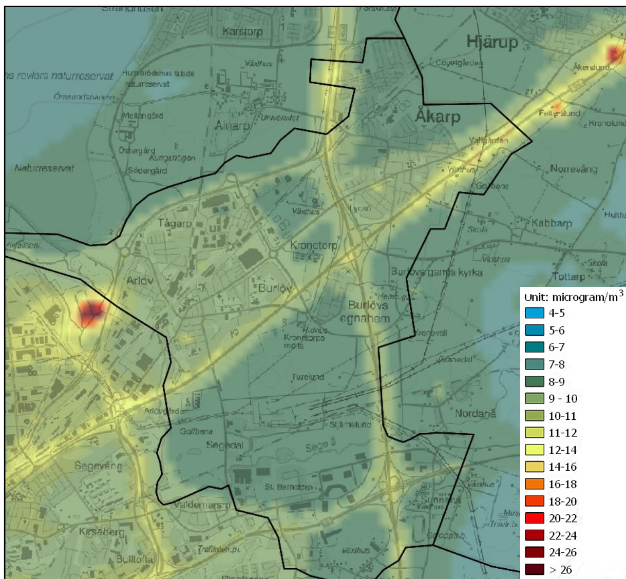
Figur 22. Beräknade årsmedelvärden av partiklar PM 2.5 inom kommunen (µg/m 3 ).
