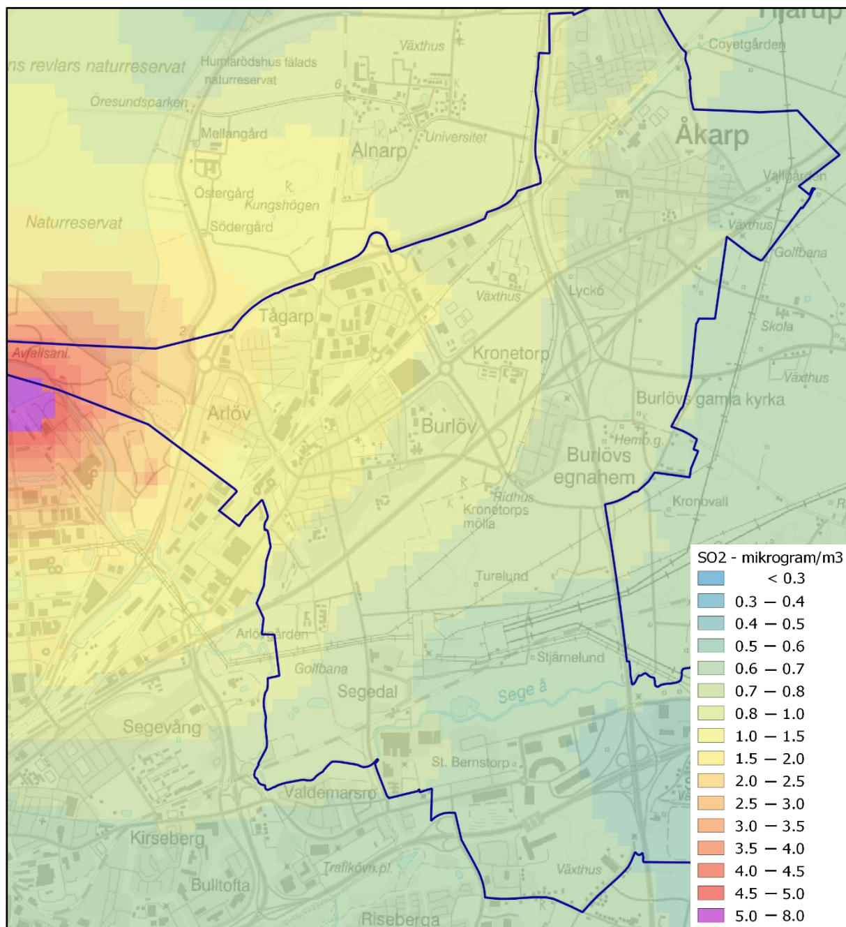
Figur 27. Beräknade årsmedelvärden av svaveldioxid ( \text{SO}_2 ) inom kommunen ( \mu\text{g}/\text{m}^3 ).
