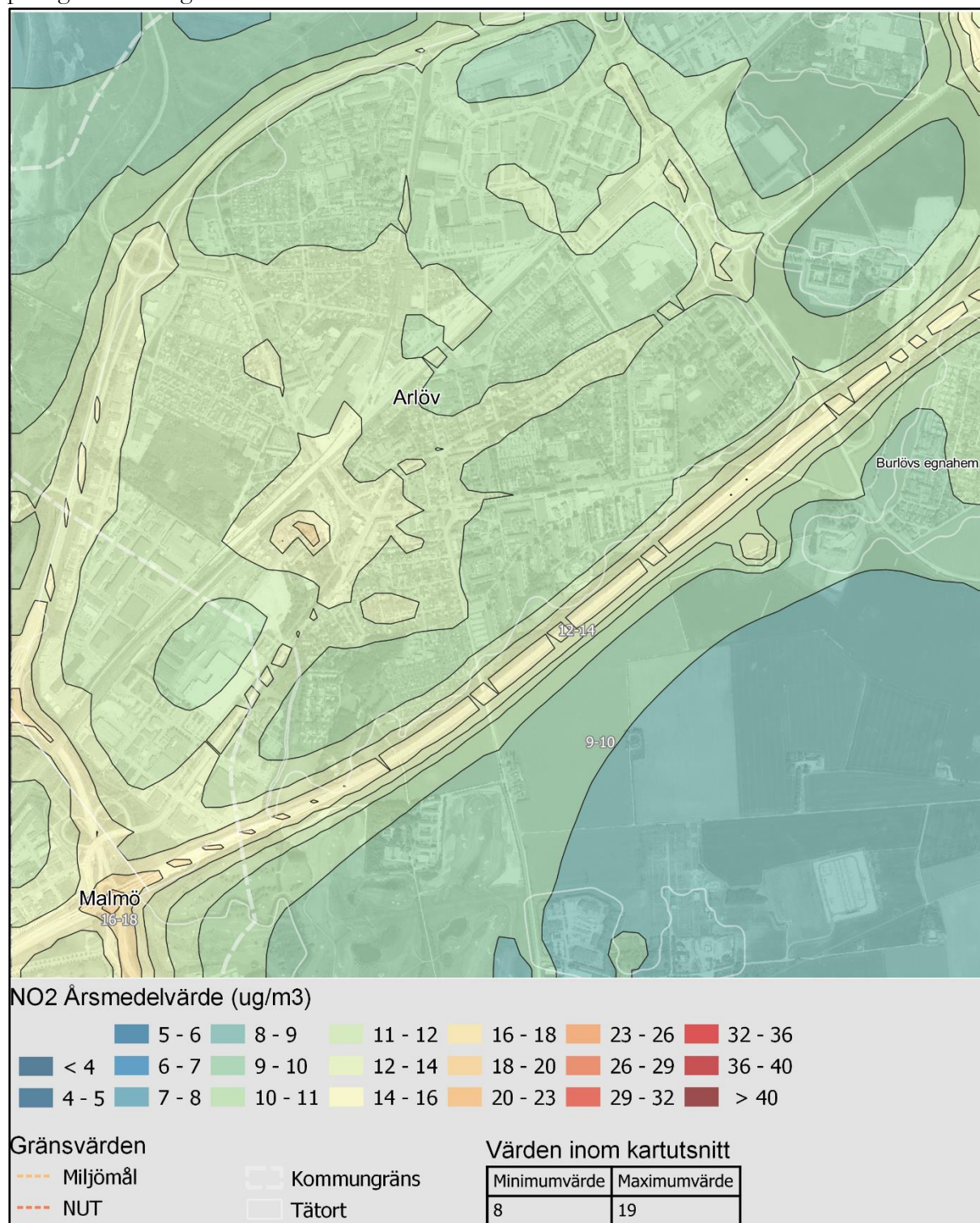
Figur 6. Beräknade årsmedelvärden av kvävedioxid i tätorten (µg/m 3 ).
