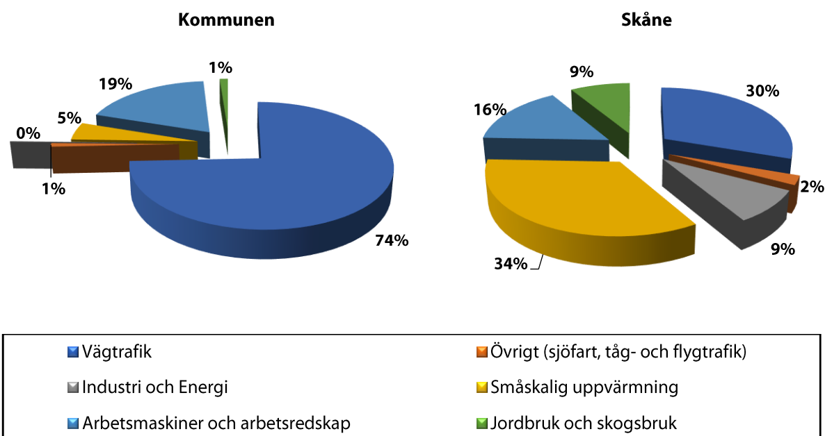
Figur 23. Procentuell fördelning av utsläppskällor för partiklar (PM 2,5 ) i kommunen jämfört med Skåne.
