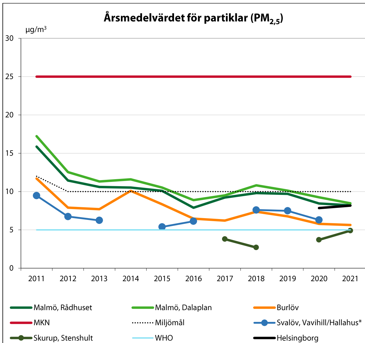
Figur 20. Årsmedelvärdet för partiklar (PM 2,5 ) under tio år inom samverkansområdet Skåne. *Mätdata saknas för 2021.
