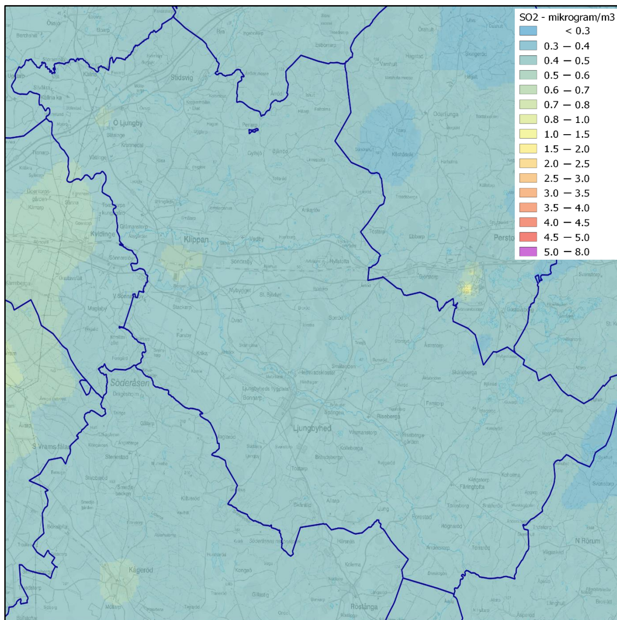
Figur 27. Beräknade årsmedelvärden av svaveldioxid ( \text{SO}_2 ) inom kommunen ( \mu\text{g}/\text{m}^3 ).
