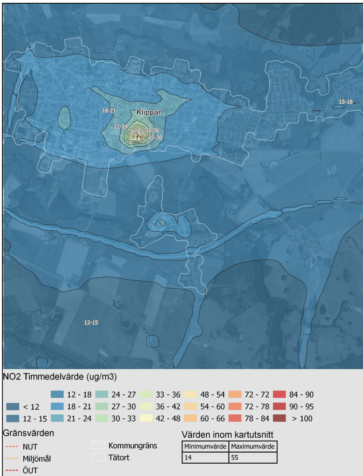
Figur 10. Beräknade timmedelvärden av kvävedioxid i tätorten ( \mu\text{g}/\text{m}^3 ).
