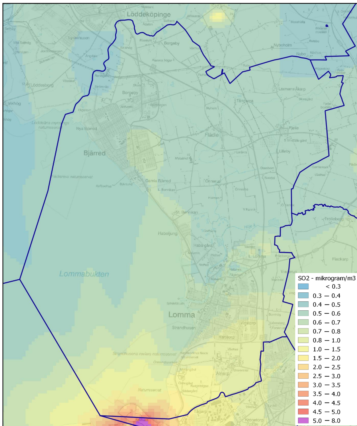
Figur 27. Beräknade årsmedelvärden av svaveldioxid ( \text{SO}_2 ) inom kommunen ( \mu\text{g}/\text{m}^3 ).
