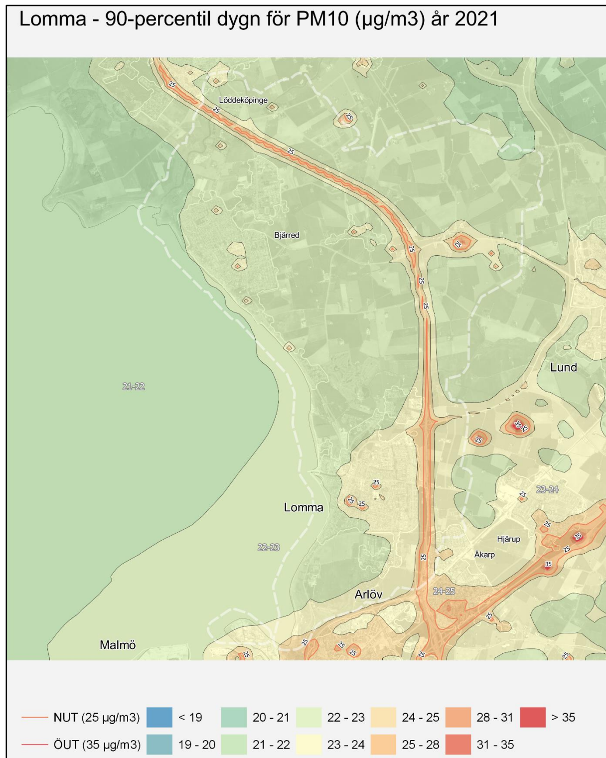
Figur 18. Beräknade dygnsmedelvärden av partiklar PM_{10} inom kommunen ( \mu\text{g}/\text{m}^3 ).
