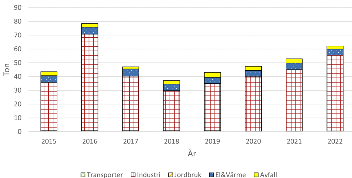
Figur 6. Visar utsläppskällorna av SO x för Eslöv, beräknat värde från SMHI.
