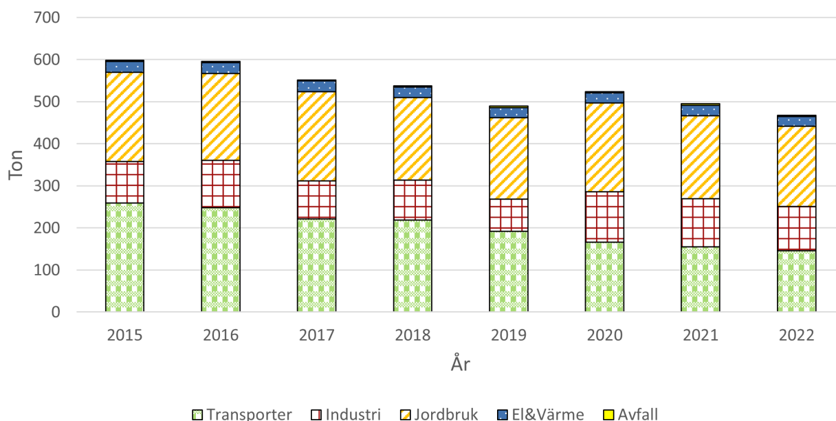
Figur 4. Visar utsläppskällorna av NO x för Eslöv, beräknat värde från SMHI.
