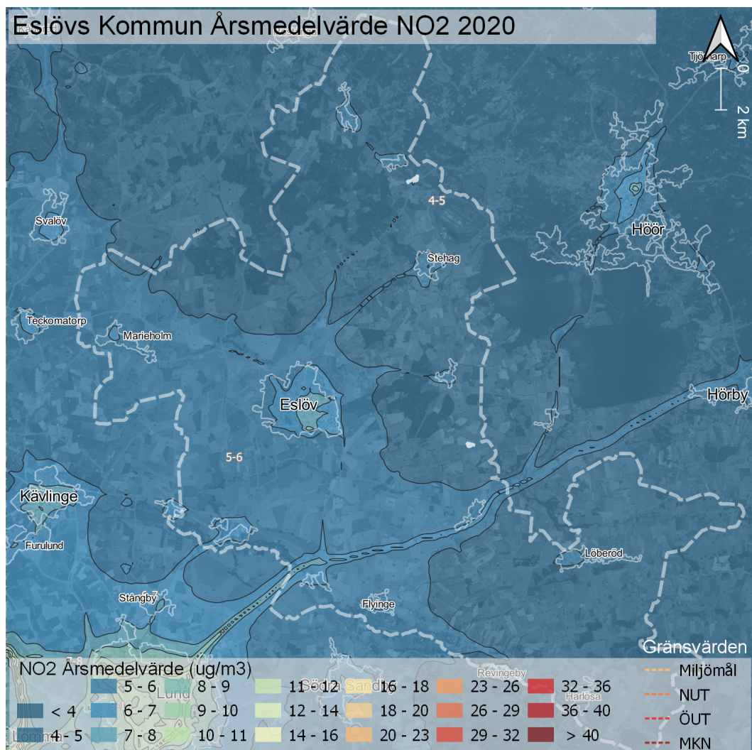
Figur 3. Karta som visar årsmedelvärden av NO 2 för år 2020 i Eslövs kommun.
