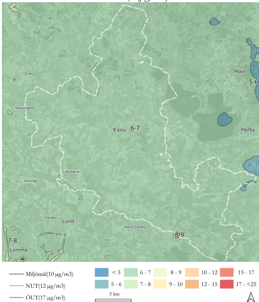
Figur 11. Karta som visar årsmedelvärdet av PM2.5 för år 2022 i Eslöv.
