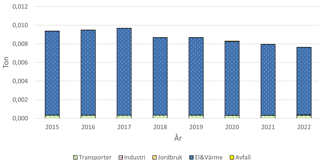
Figur 18. Visar utsläppskällorna av PAH för Eslöv, vilket inkluderar bens(a)pyren. beräknat värde från SMHI.
