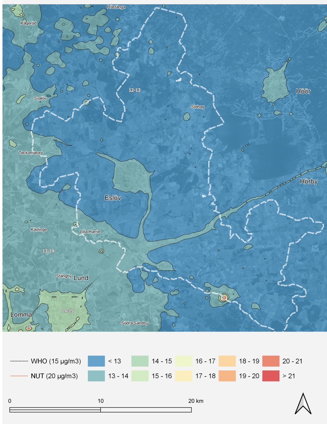
Figur 8. Karta som visar årsmedelvärdet av PM10 för år 2021 i Eslöv.
