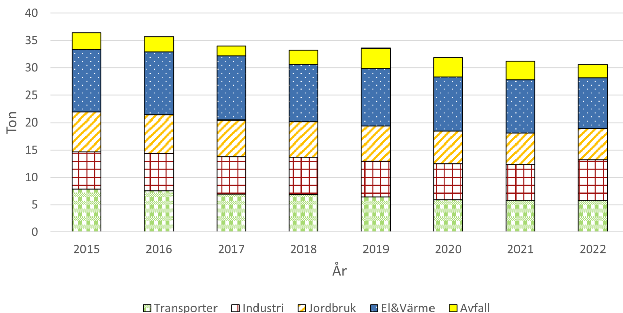
Figur 12. Visar utsläppskällorna av PM2.5 för Eslöv, beräknat värde från SMHI.
