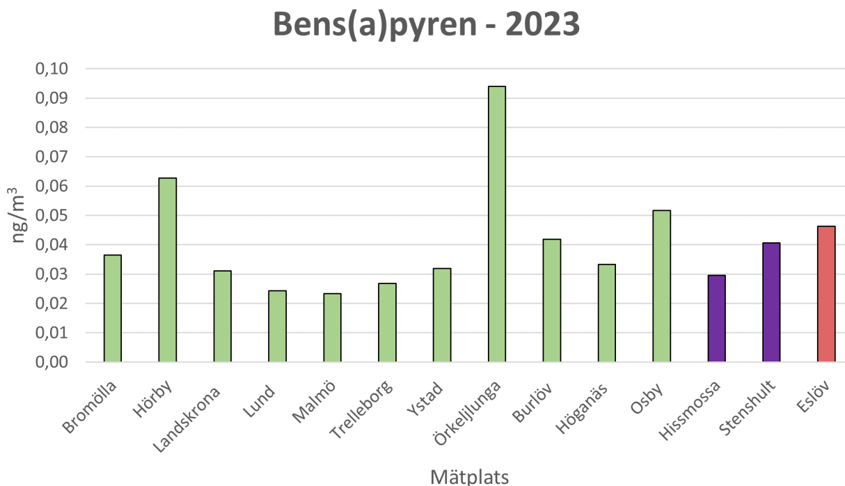
Figur 17. Visar hur medelkoncentrationen av bens(a)pyren i atmosfären såg ut i elva kommuner, två bakgrundstationer samt ett skattat värde för Eslöv i Skåne under en tremånaders mätkampanj i 2023.
