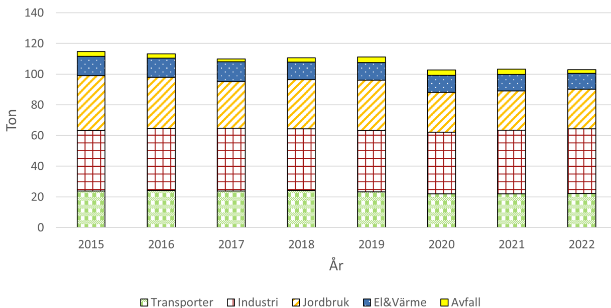
Figur 9. Visar utsläppskällorna av PM10 för Eslöv, beräknat värde från SMHI.
