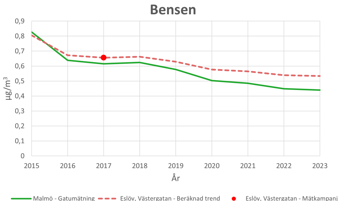
Figur 19. Visar hur koncentrationen av bensen i atmosfären har förändrats för år 2015 – 2023 i Eslöv jämfört med Malmö.
