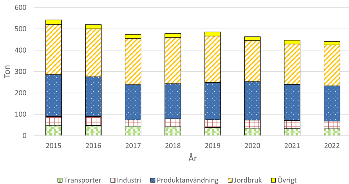
Figur 20. Visar utsläppskällorna av VOC för Eslöv, beräknat värde från SMHI.
