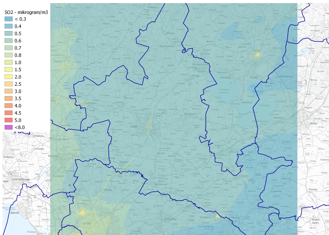
Figur 6. Karta som visar årsmedelvärden av SO x för år 2019 i Eslöv.
