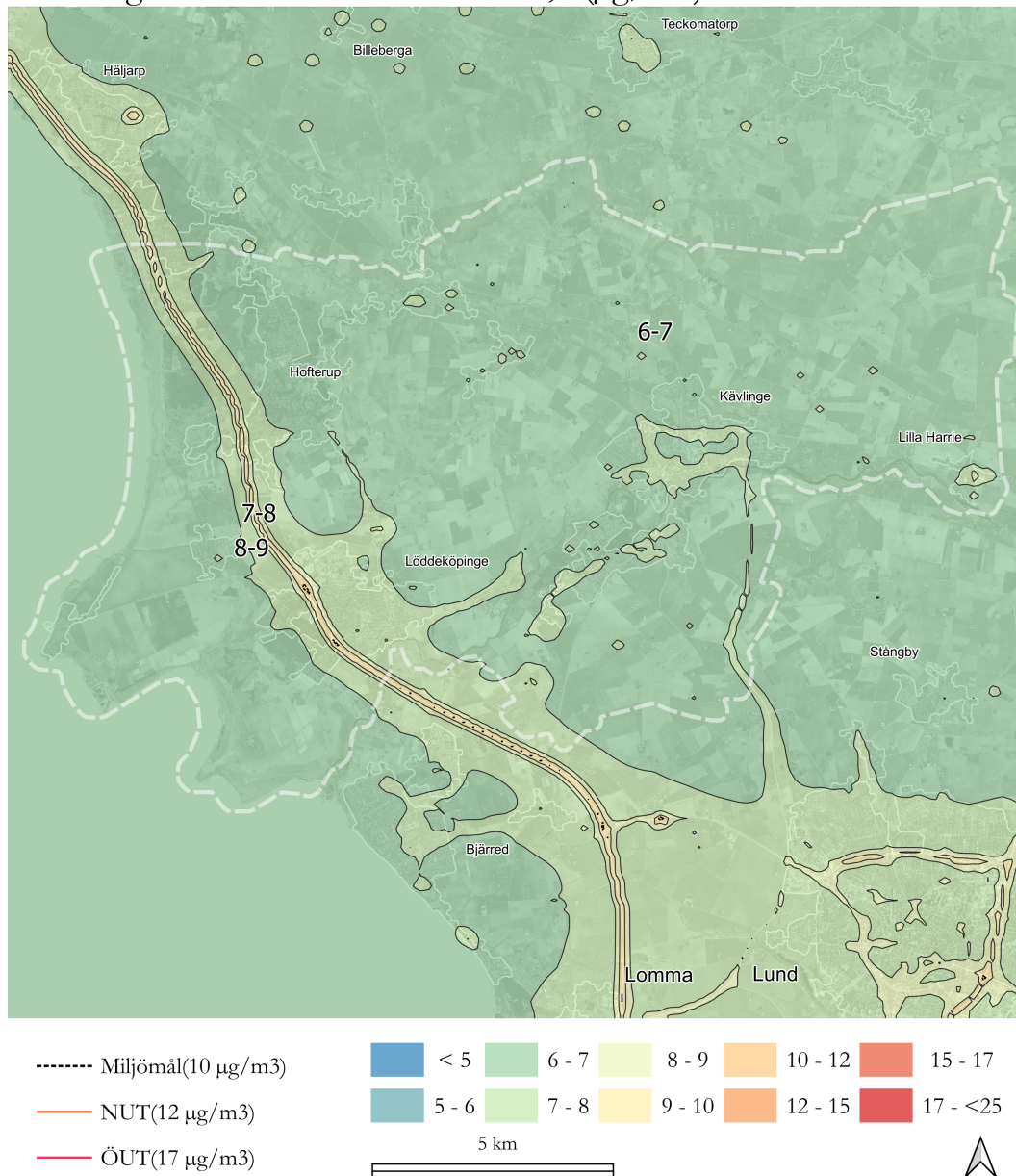
Figur 11. Karta som visar årsmedelvärdet av PM2.5 för år 2022 i Kävlinge.
