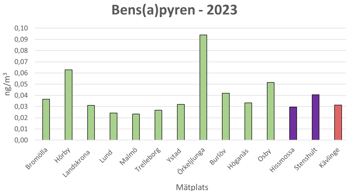
Figur 17. Visar hur medelkoncentrationen av bens(a)pyren i atmosfären såg ut i elva kommuner, två bakgrundstationer samt ett skattat värde för Kävlinge i Skåne under en tremånaders mätkampanj i 2023.
