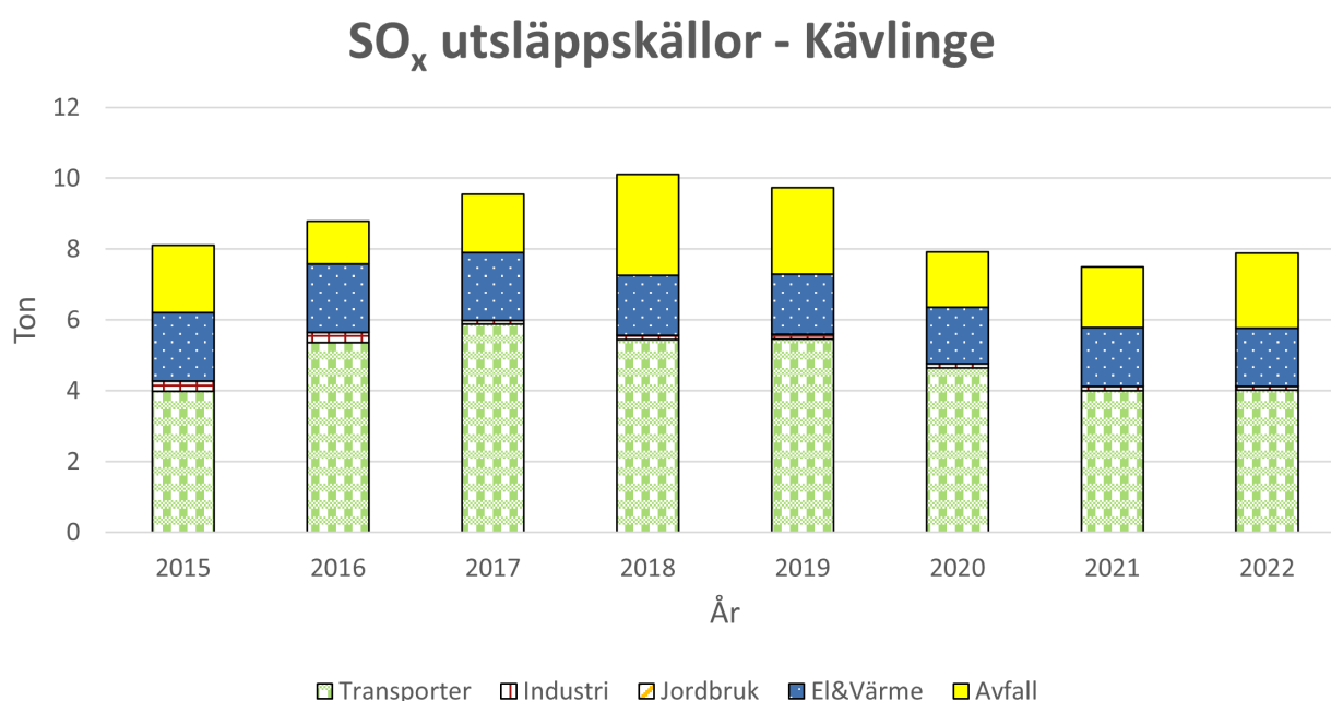
Figur 6. Visar utsläppskällorna av SO x för Kävlinge, beräknat värde från SMHI.
