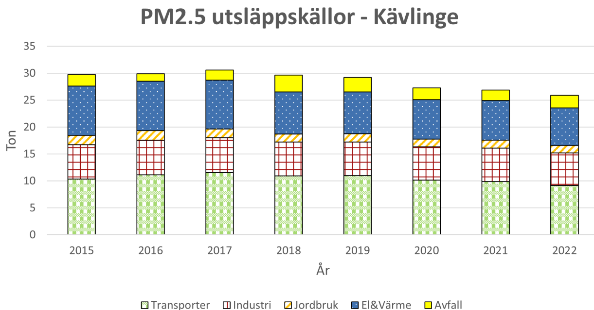
Figur 12. Visar utsläppskällorna av PM2.5 för Kävlinge, beräknat värde från SMHI.
