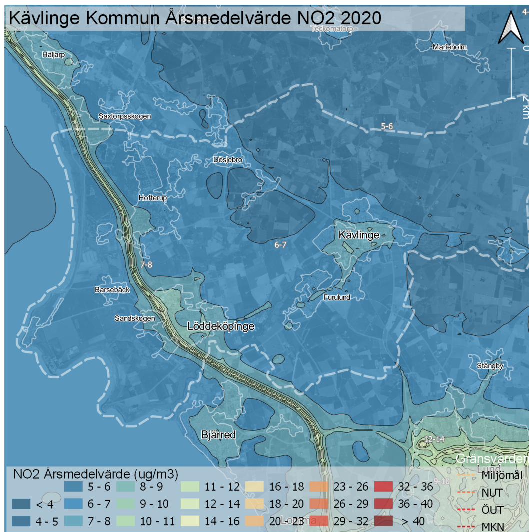
Figur 3. Karta som visar årsmedelvärden av NO 2 för år 2020 i Kävlinge kommun.
