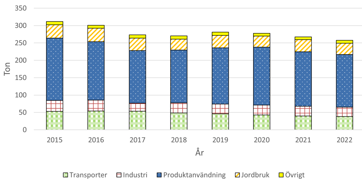
Figur 20. Visar utsläppskällorna av VOC för Kävlinge, beräknat värde från SMHI.
