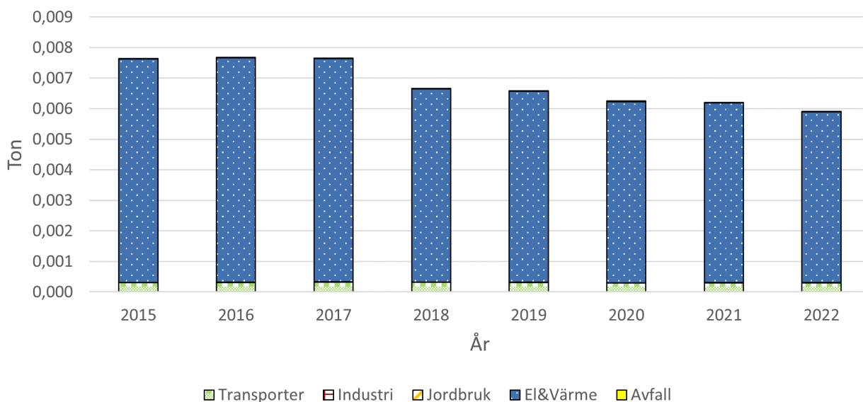
Figur 18. Visar utsläppskällorna av PAH för Kävlinge, vilket inkluderar bens(a)pyren. beräknat värde från SMHI.
