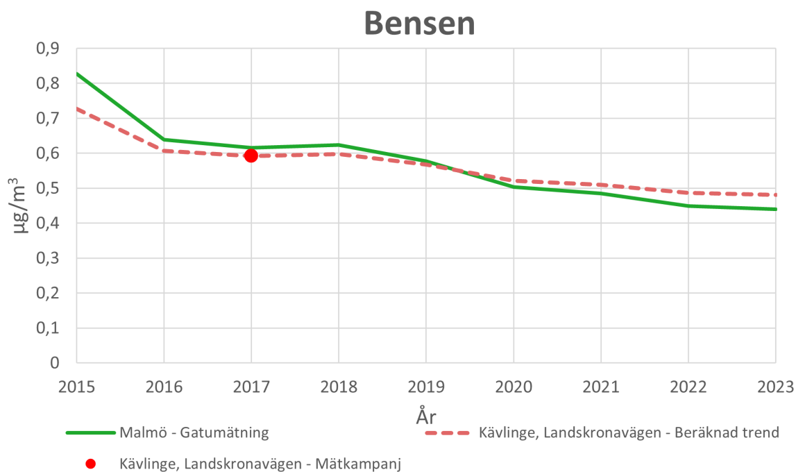
Figur 19. Visar hur koncentrationen av bensen i atmosfären har förändrats för år 2015 – 2023 i Kävlinge jämfört med Malmö.
