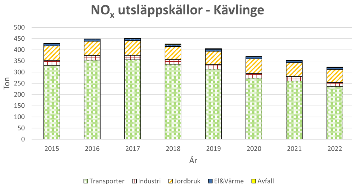
Figur 4. Visar utsläppskällorna av NO x för Kävlinge, beräknat värde från SMHI.
