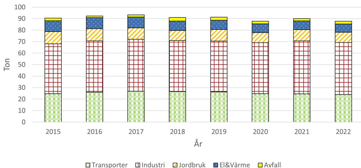
Figur 9. Visar utsläppskällorna av PM10 för Kävlinge, beräknat värde från SMHI.
