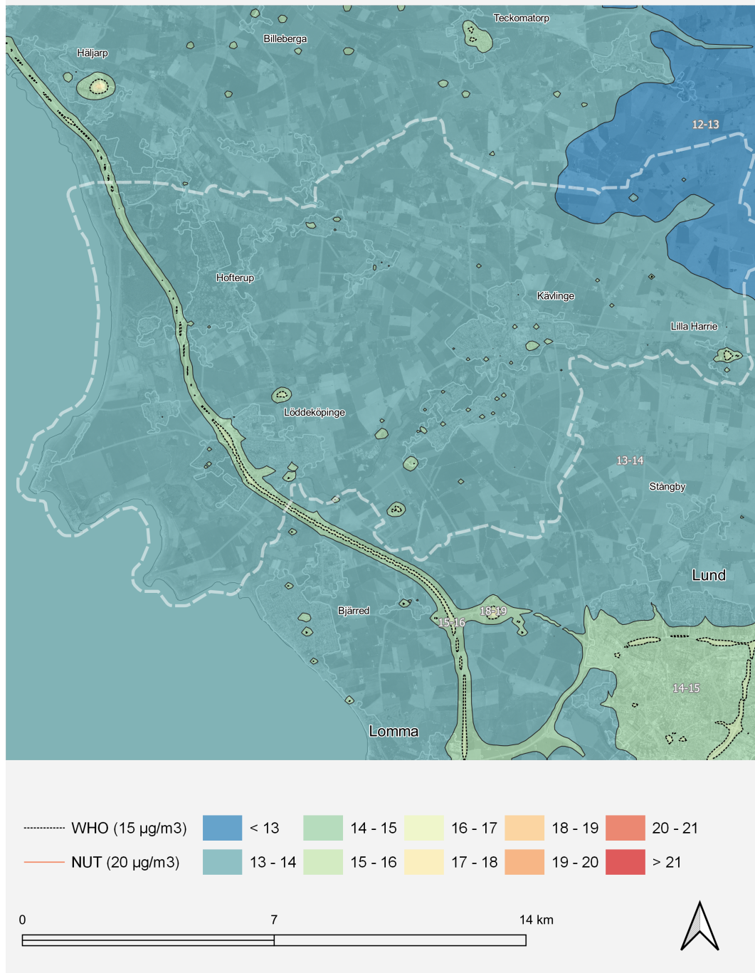
Figur 8. Karta som visar årsmedelvärdet av PM10 för år 2021 i Kävlinge.
