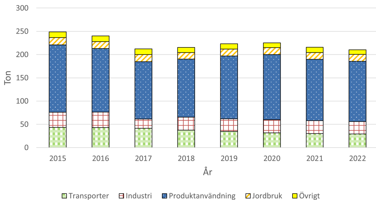
Figur 20. Visar utsläppskällorna av VOC för Staffanstorp, beräknat värde från SMHI.
