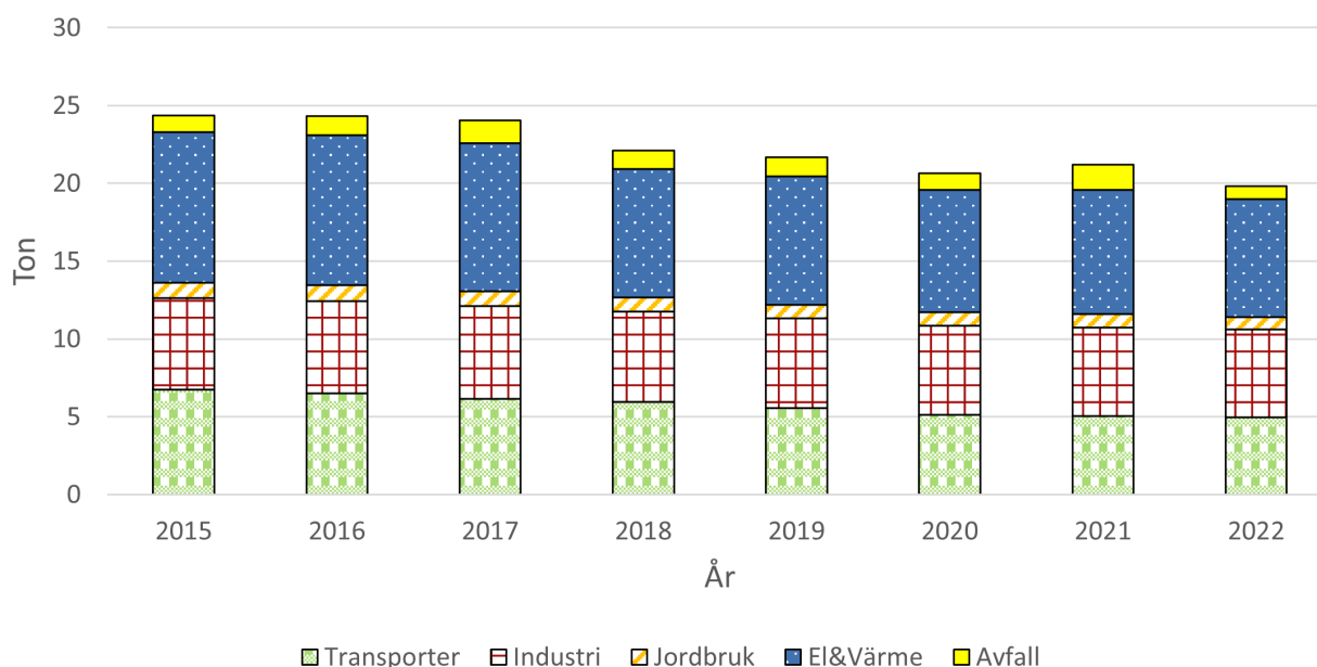
Figur 12. Visar utsläppskällorna av PM2.5 för Staffanstorp, beräknat värde från SMHI.
