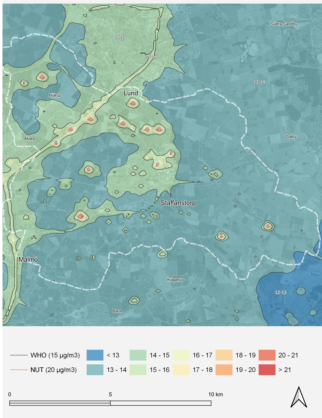
Figur 8. Karta som visar årsmedelvärdet av PM10 för år 2021 i Staffanstorp.
