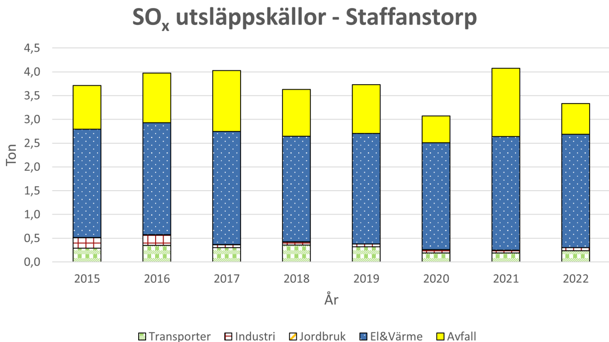
Figur 6. Visar utsläppskällorna av SO x för Staffanstorps kommun, beräknat värde från SMHI.
