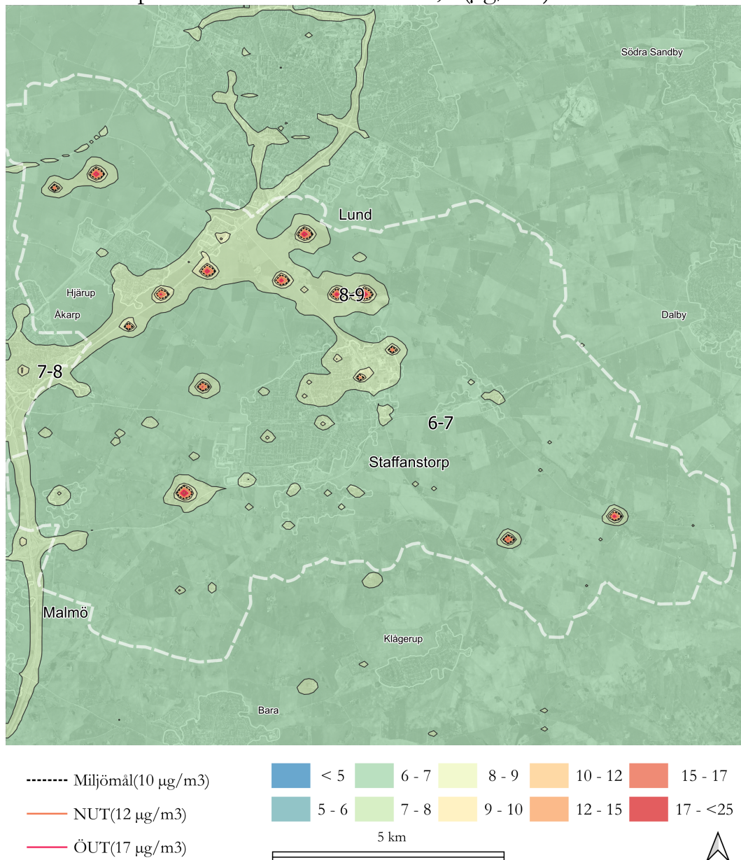
Figur 11. Karta som visar årsmedelvärdet av PM2.5 för år 2022 i Staffanstorp.
