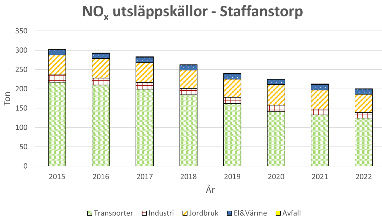
Figur 4. Visar utsläppskällorna av NO x för Staffanstorp, beräknat värde från SMHI.
