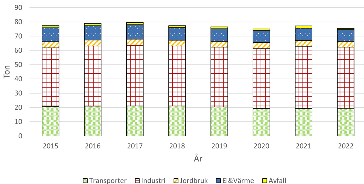
Figur 9. Visar utsläppskällorna av PM10 för Staffanstorp, beräknat värde från SMHI.
