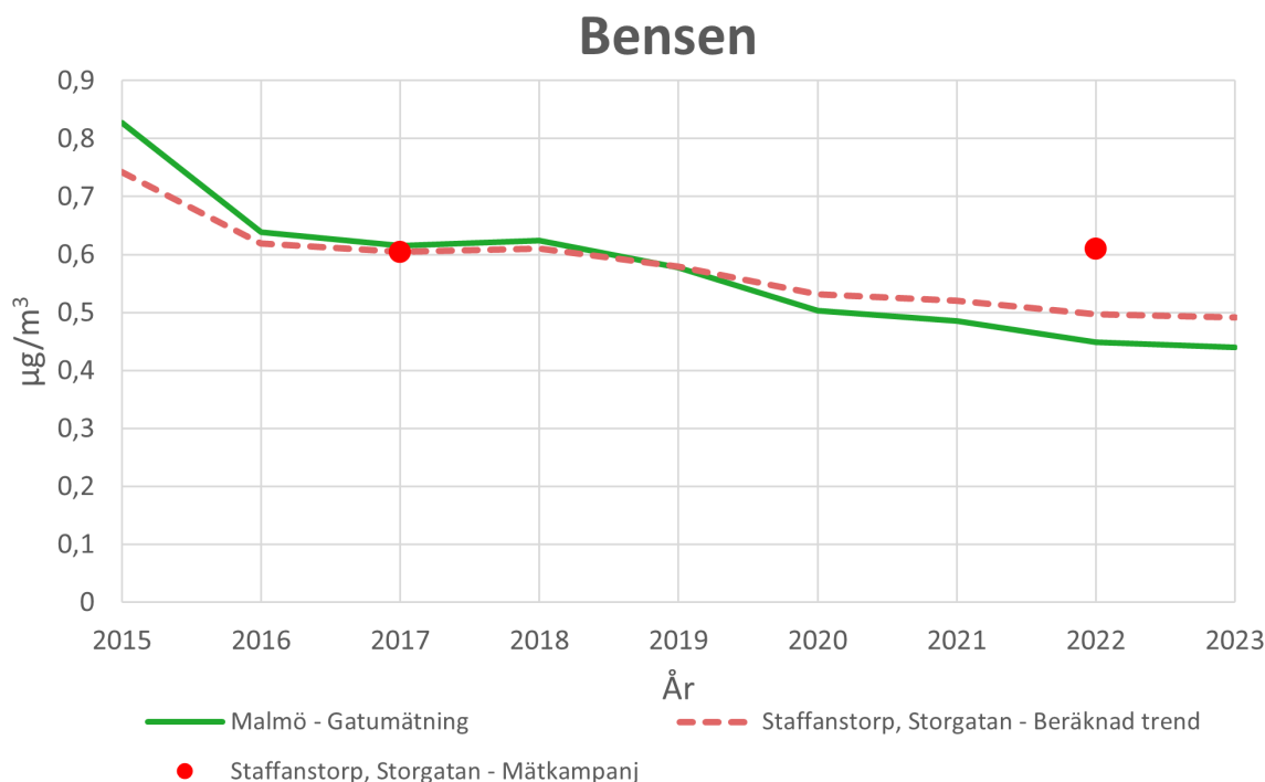
Figur 19. Visar hur koncentrationen av bensen i atmosfären har förändrats för år 2015 – 2023 i Staffanstorp jämfört med Malmö.
