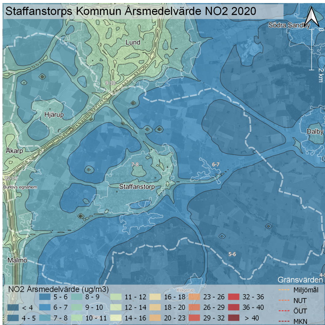
Figur 3. Karta som visar årsmedelvärden av NO 2 för år 2020 i Staffanstorps kommun.
