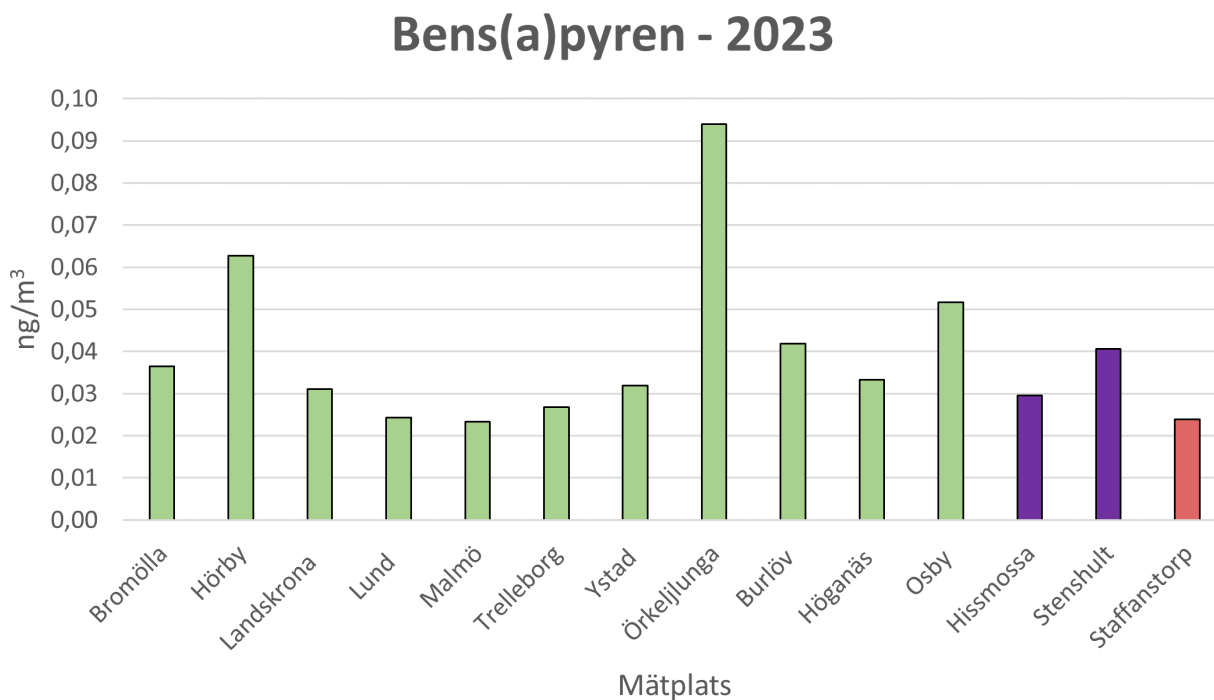
Figur 17. Visar hur medelkoncentrationen av bens(a)pyren i atmosfären såg ut i elva kommuner, två bakgrundstationer samt ett skattat värde för Staffanstorp i Skåne under en tremånaders mätkampanj i 2023.
