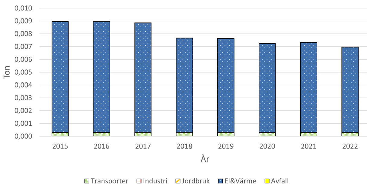
Figur 18. Visar utsläppskällorna av PAH för Staffanstorp, vilket inkluderar bens(a)pyren. beräknat värde från SMHI.
