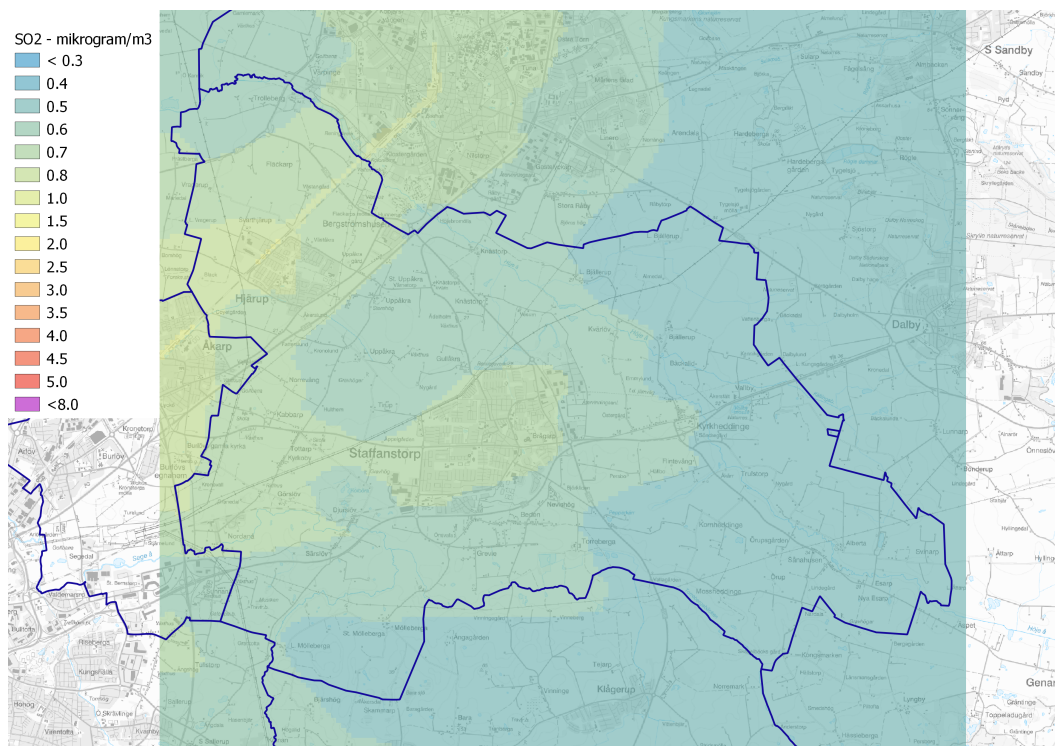
Figur 6. Karta som visar årsmedelvärde av SO x för år 2019 i Staffanstorps kommun.
